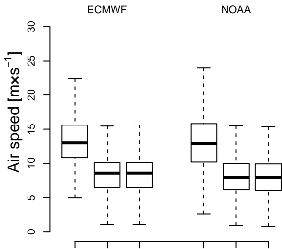
Ciconia ciconia
