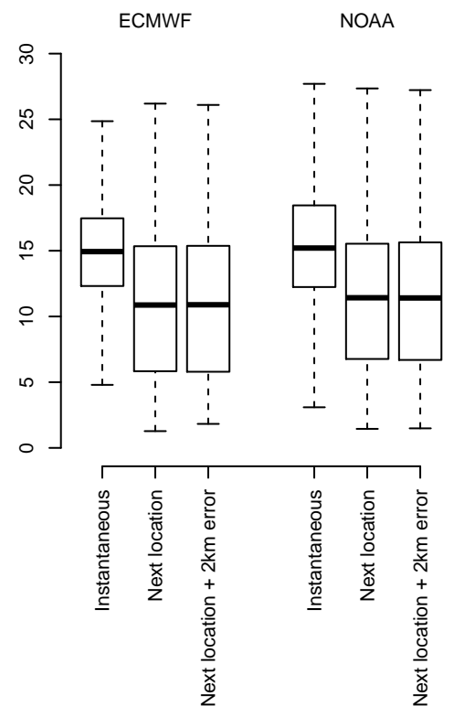
Tadorna ferruginea
