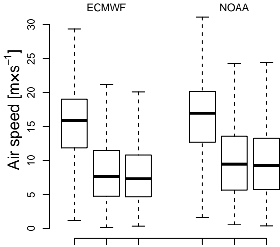
Anas platyrhynchos
