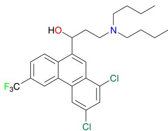
halofantrine (5)
