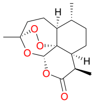
artemisinin (8)
