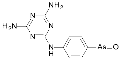
Melarsen oxid
