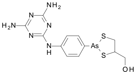
Melarsoprol
