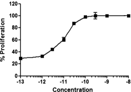
Estradiol
