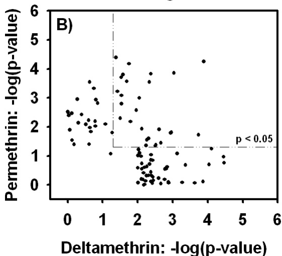
SAM Regression
