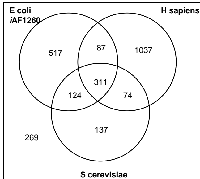
b) Metabolites
